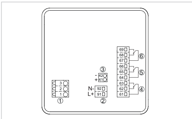
Připojovací plán VEGAMET 341
